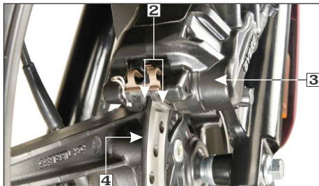
(2) ब्रेक पैड
