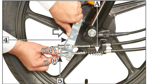
(4) इंटीग्रेटेड ब्रेक आर्म
