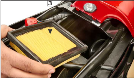
(3) एयर क्लीनर एलिमेंट
