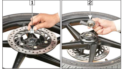
(1) साइड कॉलर
