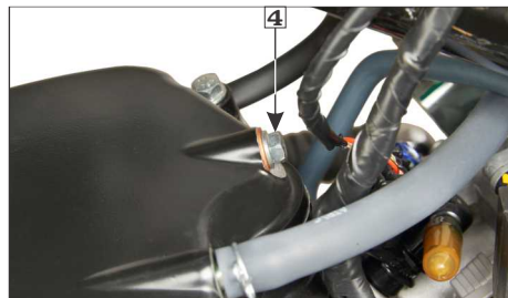
(4) इंजन ऑयल चेक बोल्ट
