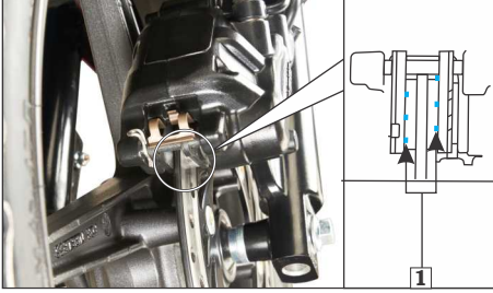
(1) वियर इंडिकेटर यूव
