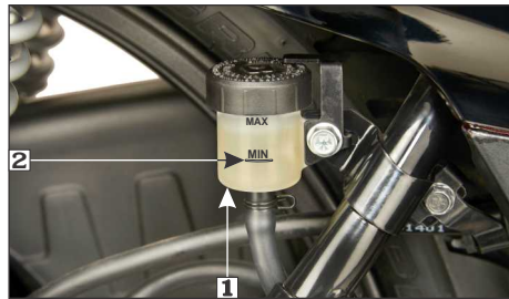
(1) रिजर्वॉयर
