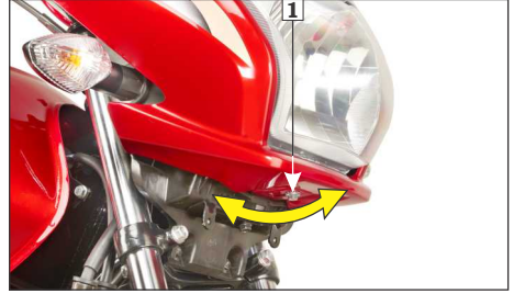
(1) हेडलैंप एडजस्टिंग बोल्ट
