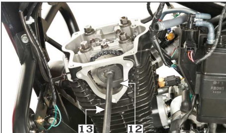
(12) कैम स्प्रॉकेट
