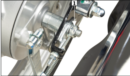
(1) रियर एक्सल नट
