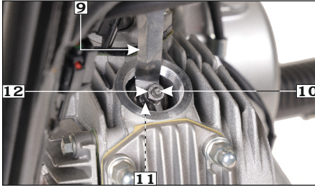
(9) फीलर गेज (10) एडजस्टिंग स्क्रू (11) वॉल्व स्टेम (12) लॉक नट
