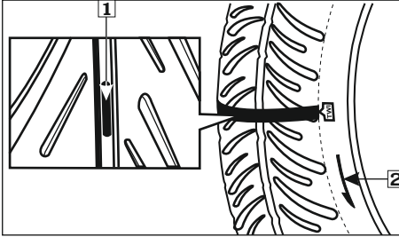
(1) वियर इंडिकेटर
