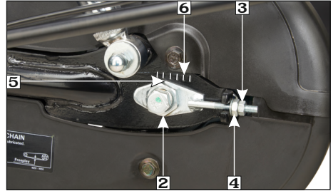
(2) स्लीव नट (3) ड्राइव चैन लॉक नट (4) ड्राइव चैन एडजस्टिंग नट (5) इंडेक्स मार्क (6) स्केल ग्रेजुएशन
